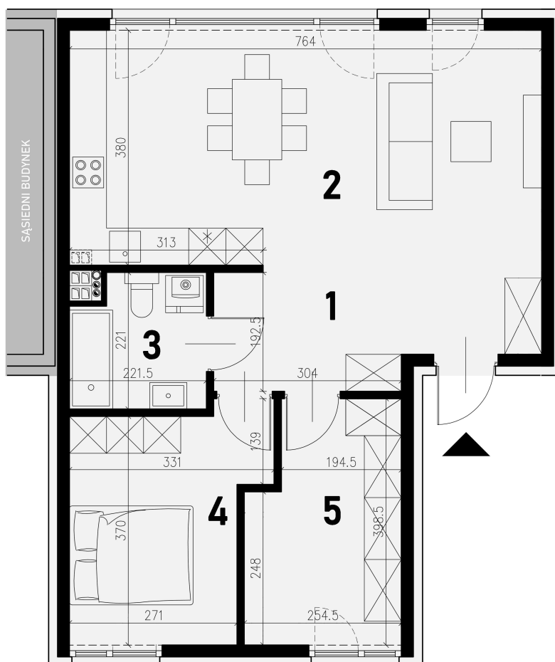
RZUT PIĘTRA
