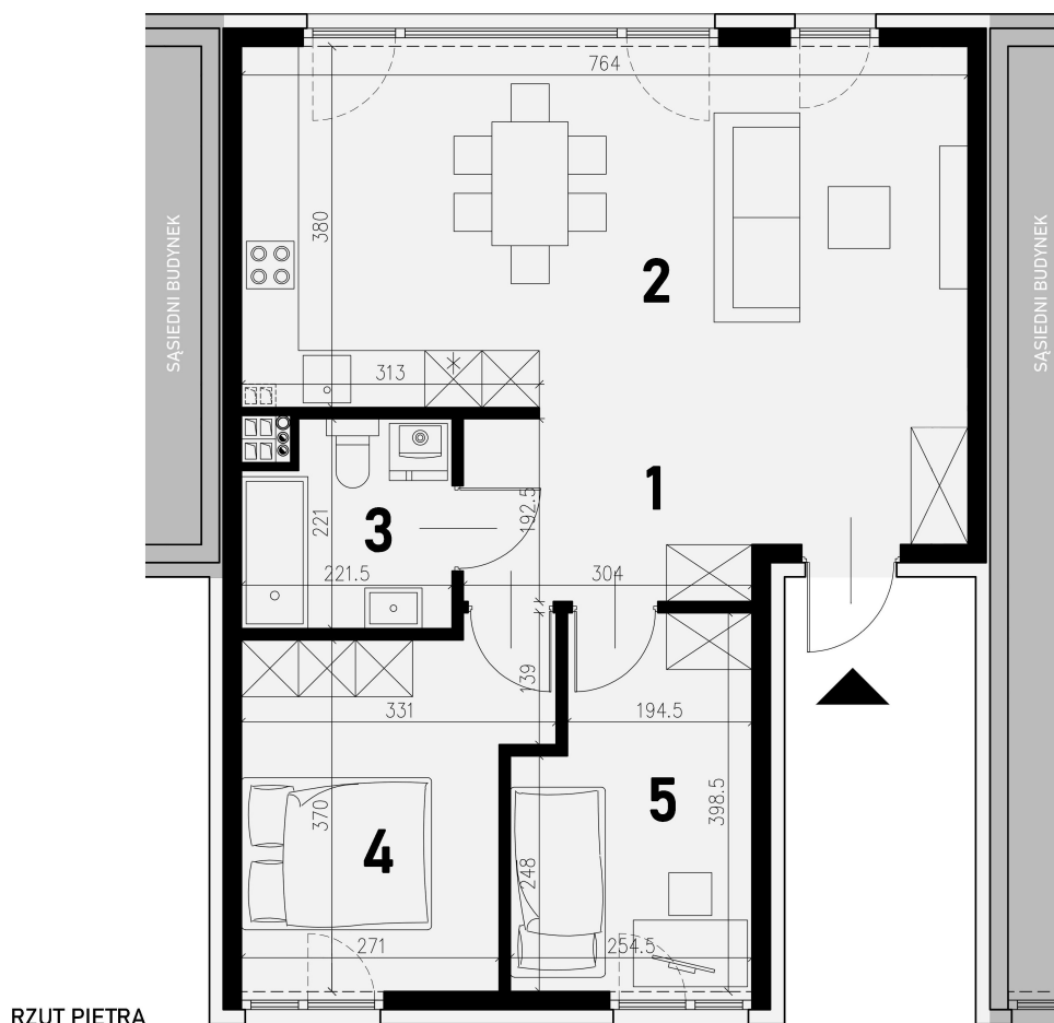
RZUT PIĘTRA
